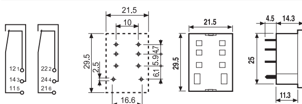
Rysunek otworów montażowych 96.12
