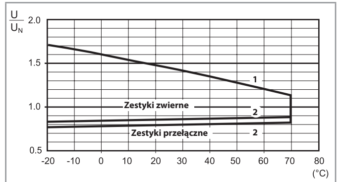
R 56 - DC Dopuszczalny zakres napięcia pracy cewki w zależności od temperatury otoczenia - 4 zestyki
