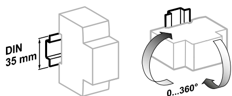
Zatrząsk na szynę DIN 35 mm. Dowlona pozycja montażu.
