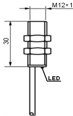
wyjście kablowe / cable output
