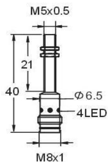
wyjście konektorowe / plug output
